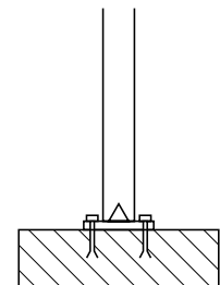
Halterung zum Aufschrauben auf Betonsockel
