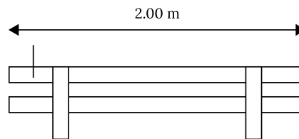
RÜCKANSICHT SITZBANK
